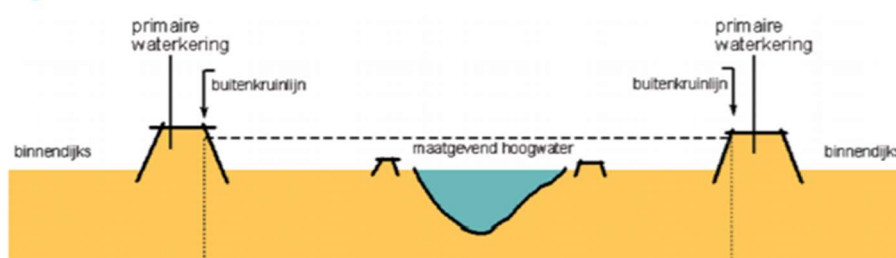
Figuur 1 Een schematische doorsnede van het rivierbed.
